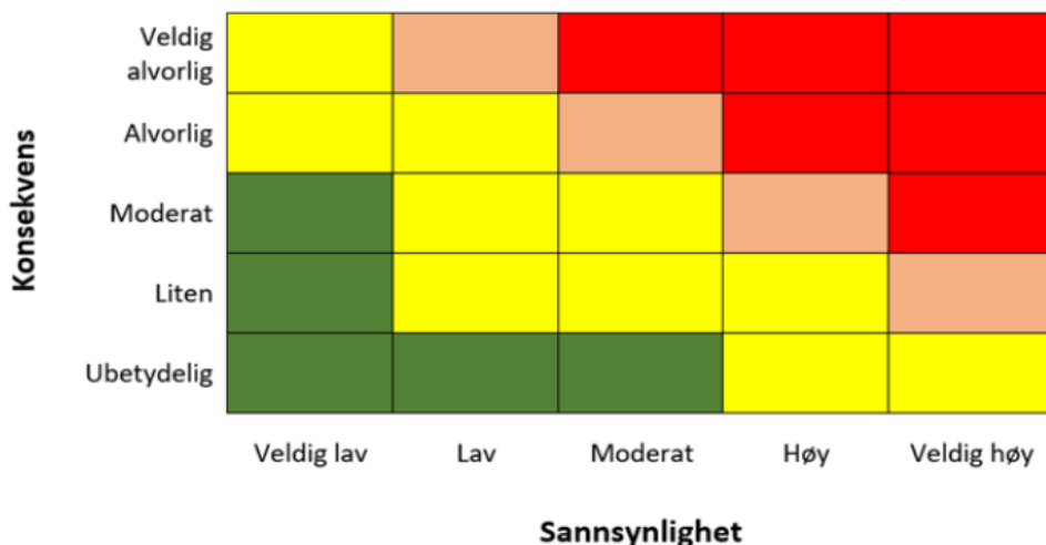
Figur 1: Risikomatrise
